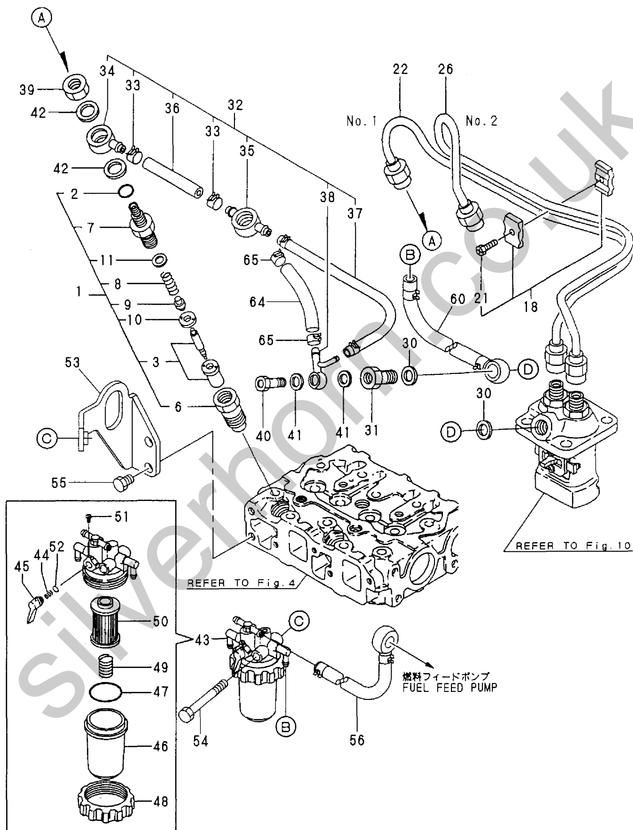
Fig. 12 燃料噴射ポンプ FUEL INJECTION PUMP
