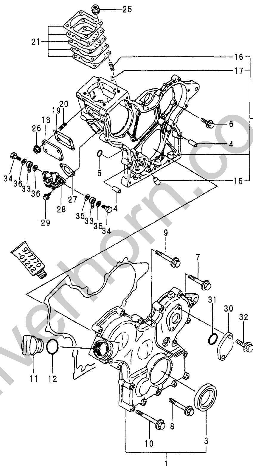
Fig. 2 ギヤケース GEAR HOUSING
