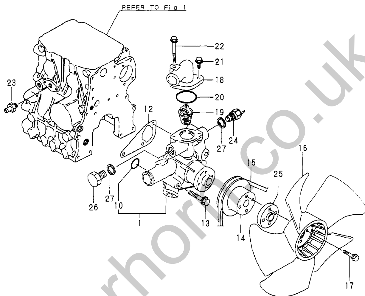
Fig. 9 冷却水システム COOLING WATER SYSTEM
