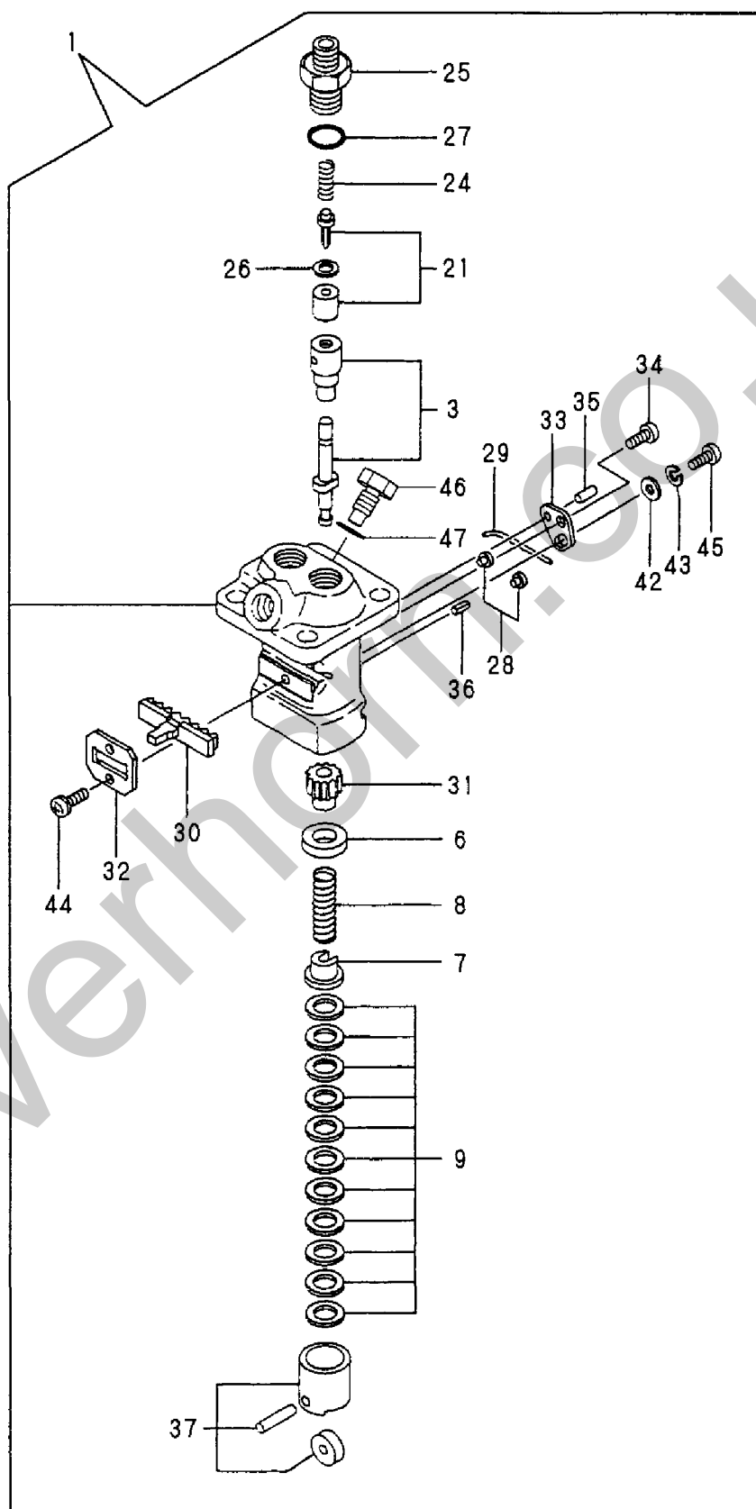
Fig. 10 燃料噴射ポンプ FUEL INJECTION PUMP
